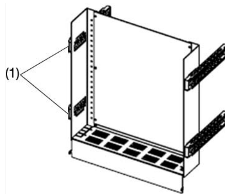
Einbau im Schrank unten (1) Befestigung ab Boden: 250 und 575 mm
