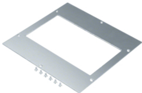
Cadre de montage 147 x 247 pour boîte de jonction acier 290 mm
