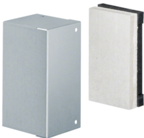
Endstück zu FWK 30 I90 50x110 verzinkt
