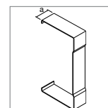
Cache-découpe Tôle en acier
