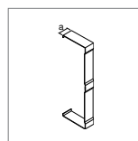
Cache-découpes Tôle en acier Cote a = 25 mm
