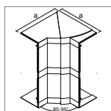
Angle intérieur réglable \pm 5^\circ PC/ABS sans halogène Cote a = 146 mm
