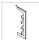
Cache-paroi Tôle en acier Cote a = 7 mm
