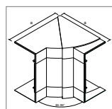
Angle intérieur réglable \pm 5^\circ PC/ABS sans halogène Cote a = 143 mm
