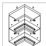
Angle intérieur Tôle en acier
