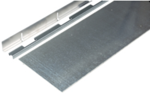
Oberteil geschlossen BKB 250x85mm L=1m
